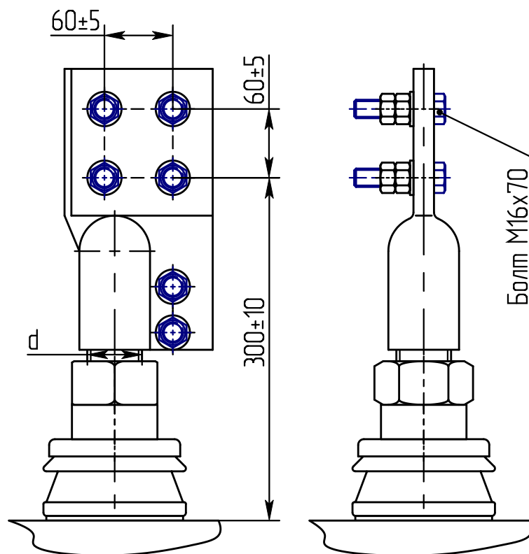
Рисунок А.18 – Ввод НН на номинальный ток 2500 А
