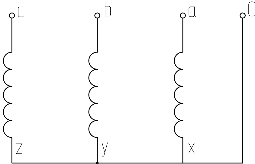
Рисунок А.26 – Схема подсоединения ответвлений обмоток НН к переключателю при схеме соединения обмоток – «ЗВЕЗДА С НУЛЕМ»
